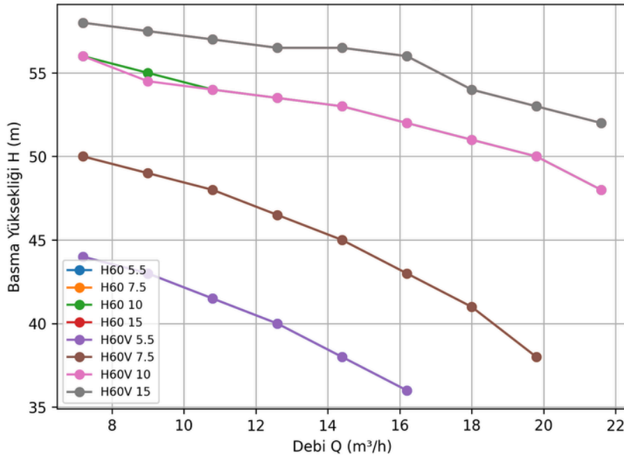
H60 / H60-V Q-H Grafiği
