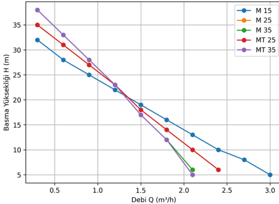
MAKSİ Q-H Grafiği
