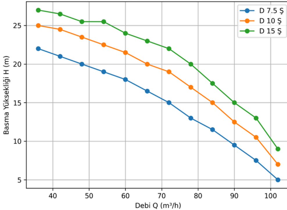
DUR Şaseli Q-H Grafiği
