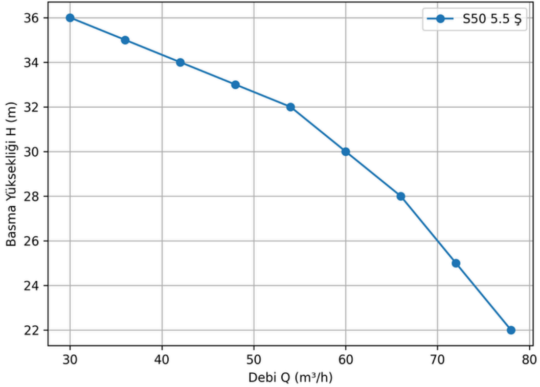
S50 Şaseli Q-H Grafiği
