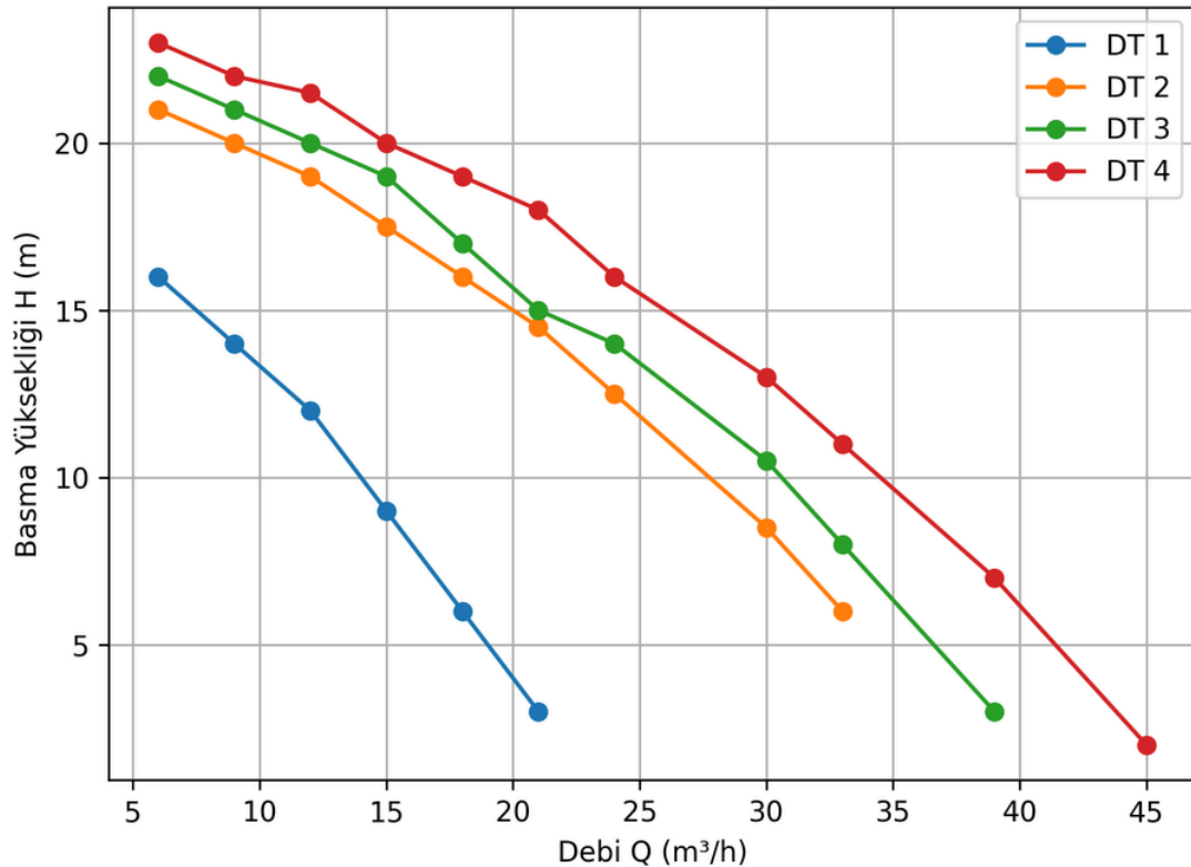
DUR Q-H Grafiği
