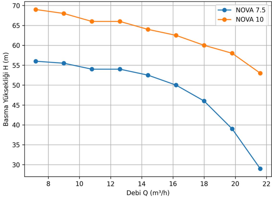
NOVA Q-H Grafiği
