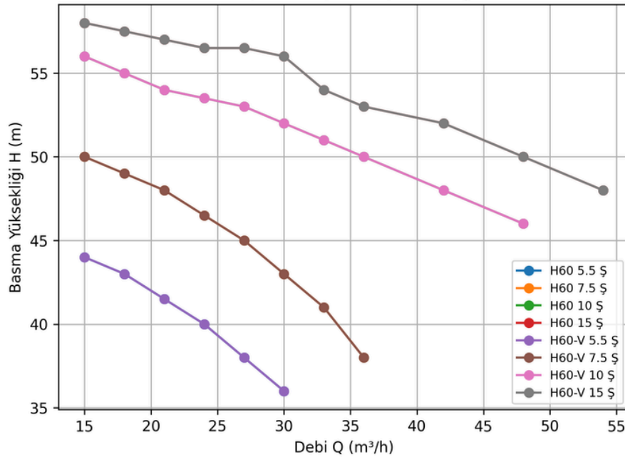
H60 / H60-V Şaseleli Q-H Grafiği
