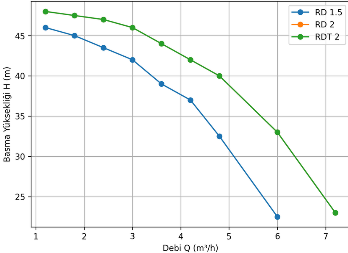
RD (2 Kademe) Q-H Grafiği
