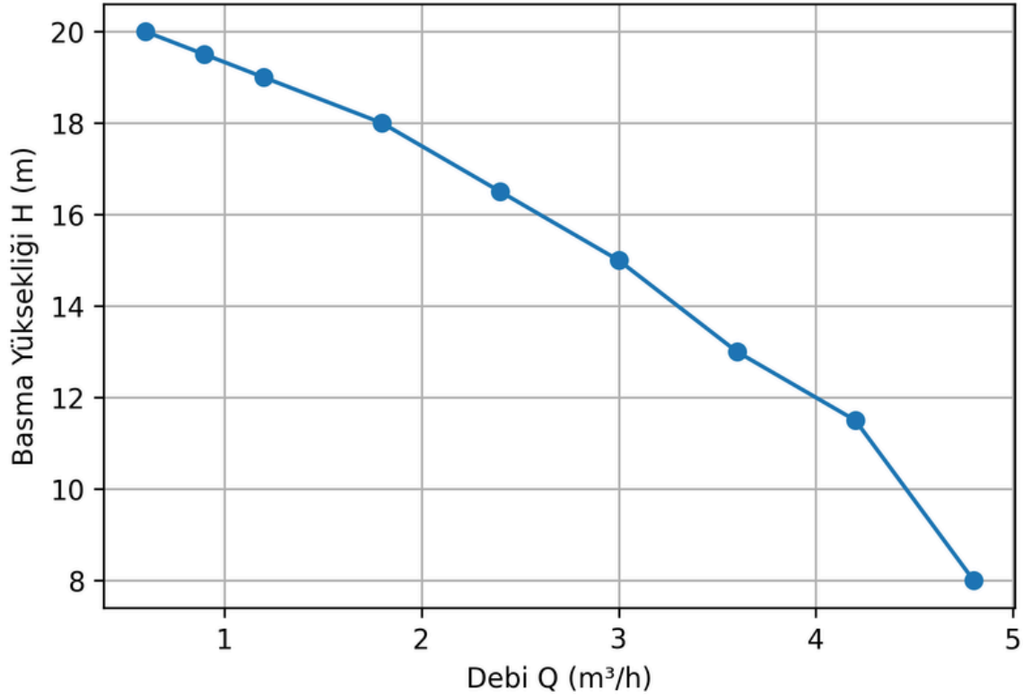
SM Q-H Grafiği
