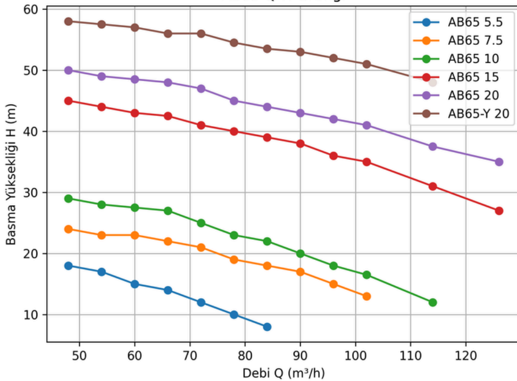
AB65 Q-H Grafiği
