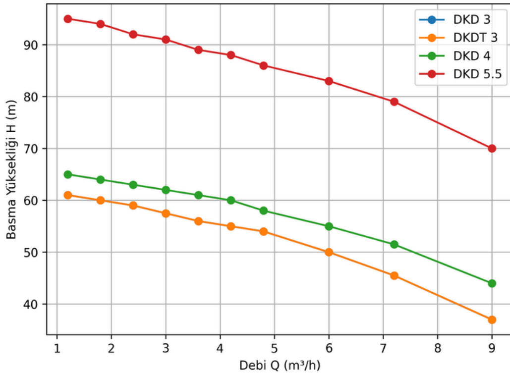
DKD Q-H Grafiği
