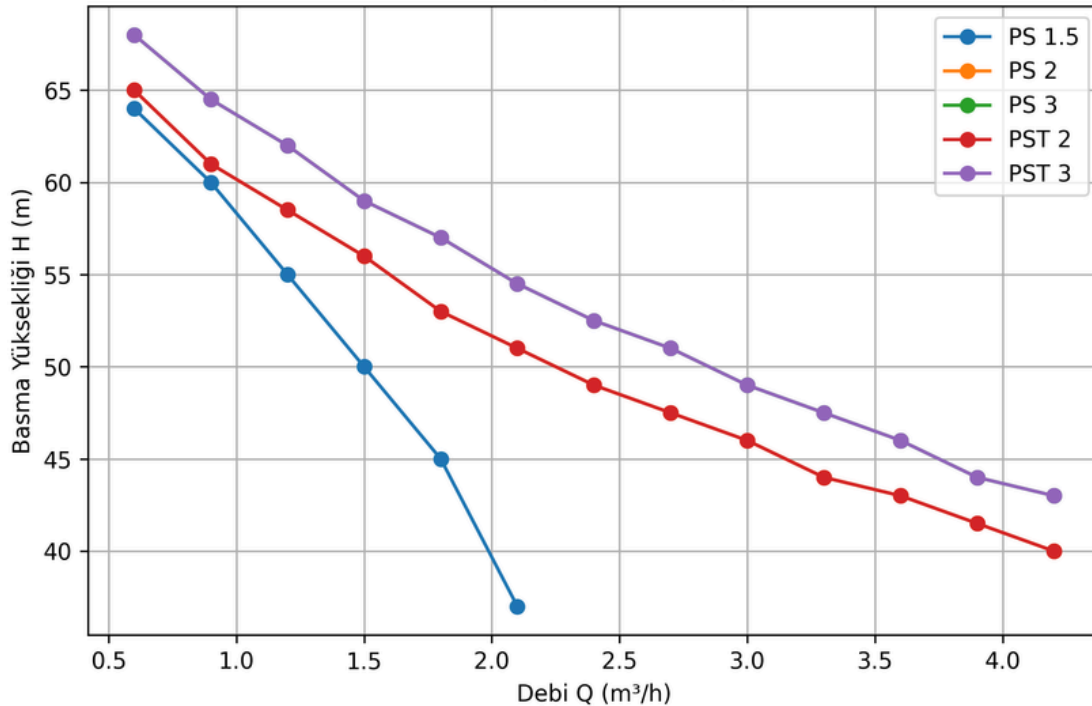
PULSA-JET Q-H Grafiği
