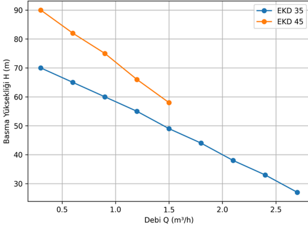
EKD Q-H Grafiği
