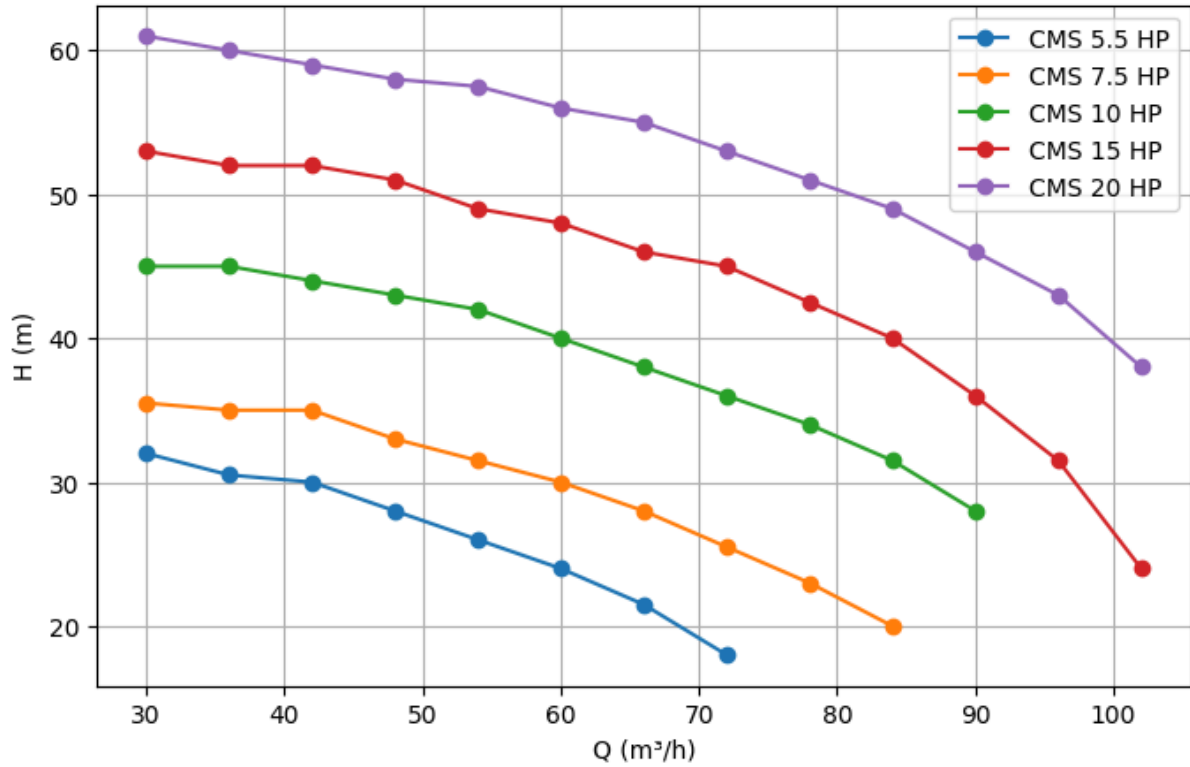
CMS Serisi Q/H Performans Eğrileri
