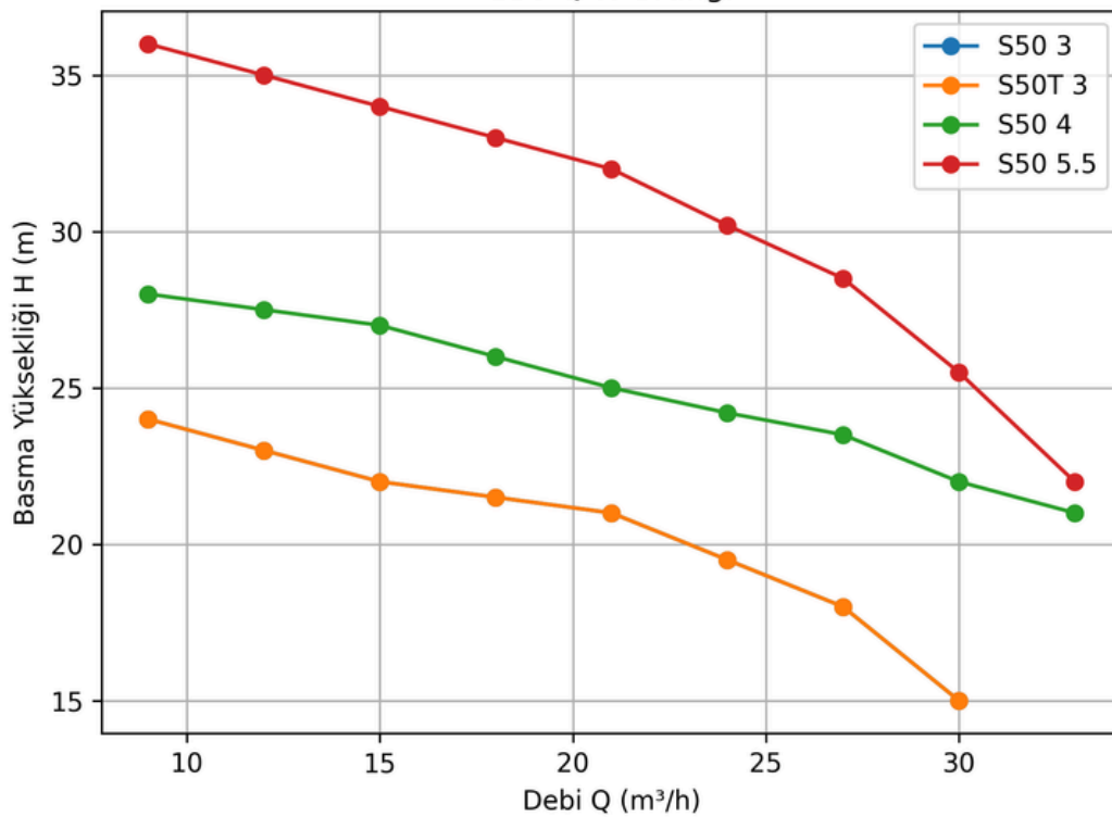
S50 Q-H Grafiği
