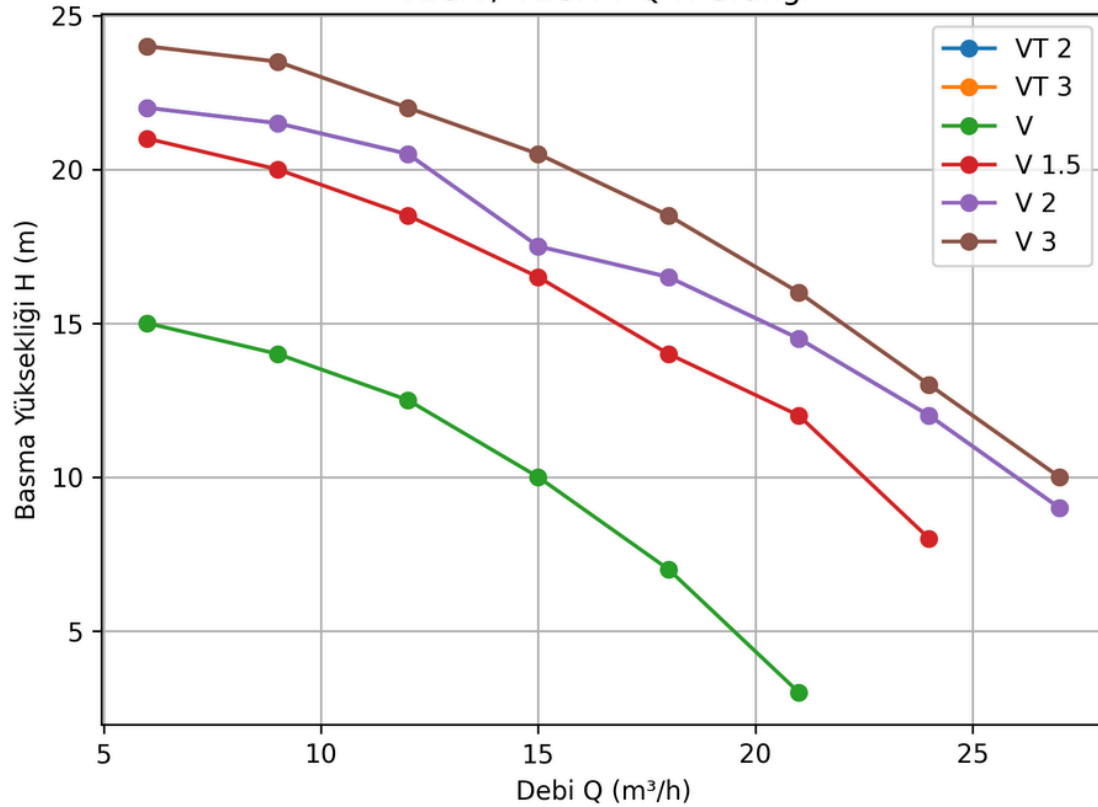
VEGA / VEGA-V Q-H Grafiği
