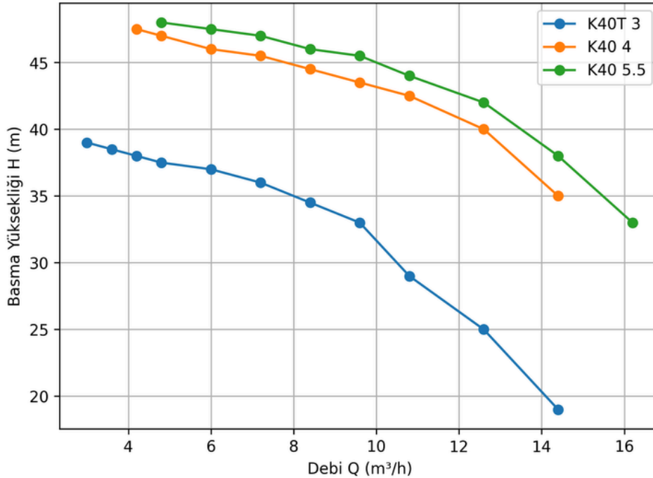
K40 Q-H Grafiği
