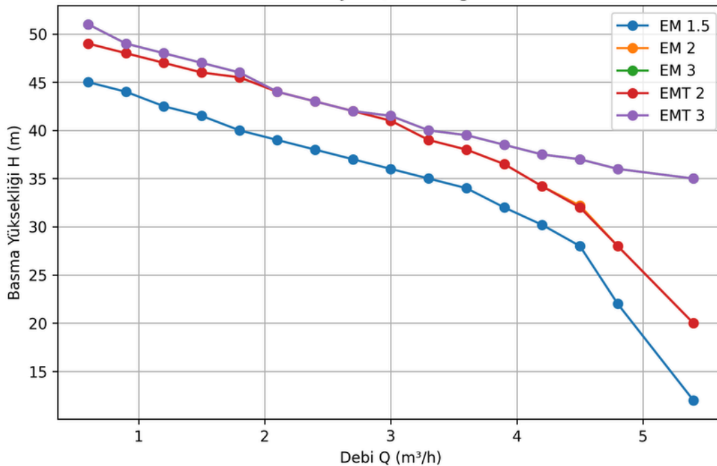
EM-JET Q-H Grafiği
