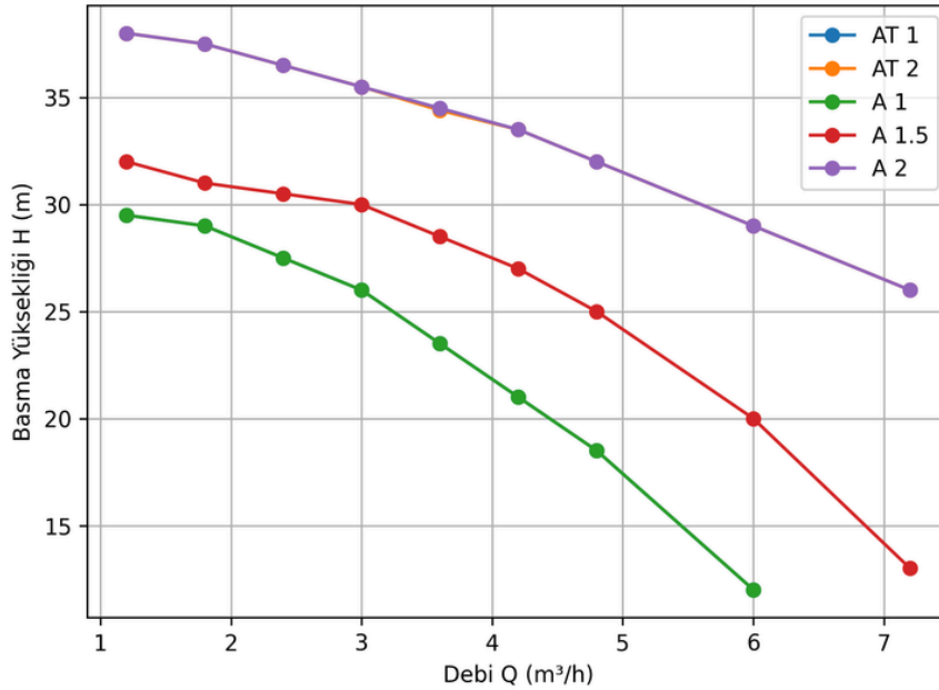
ASTRA Q-H Grafiği
