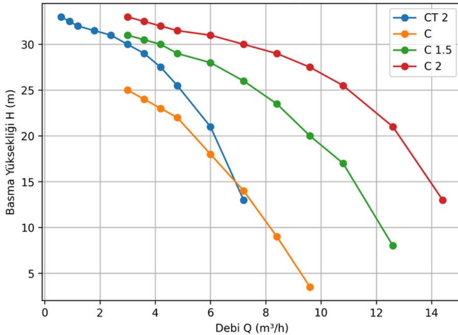
C40 Q-H Grafiği
