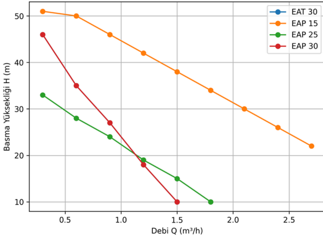
EAP / EAT Q-H Grafiği
