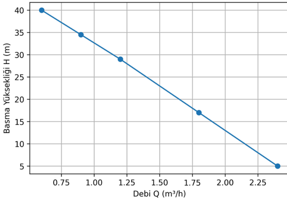
SUT / SU Q-H Grafiği
