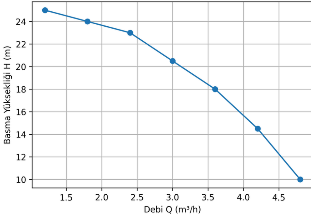
KM Q-H Grafiği
