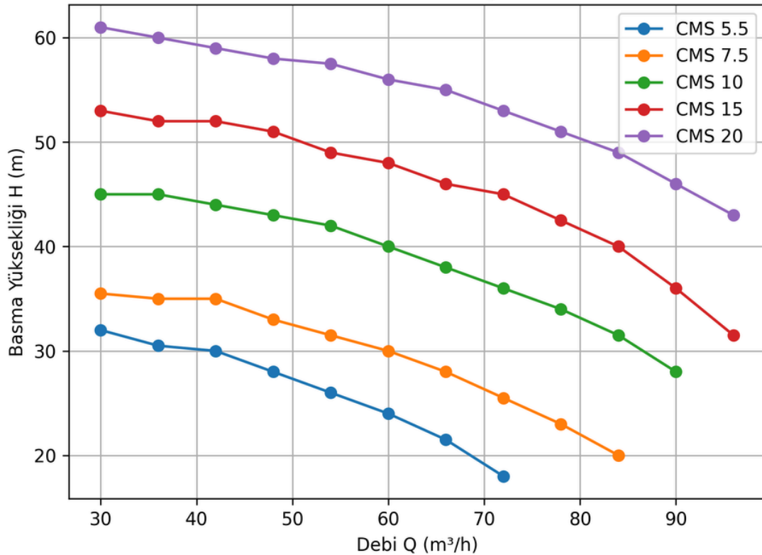
CMS Q-H Grafiği
