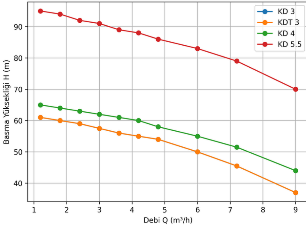
KD Q-H Grafiği
